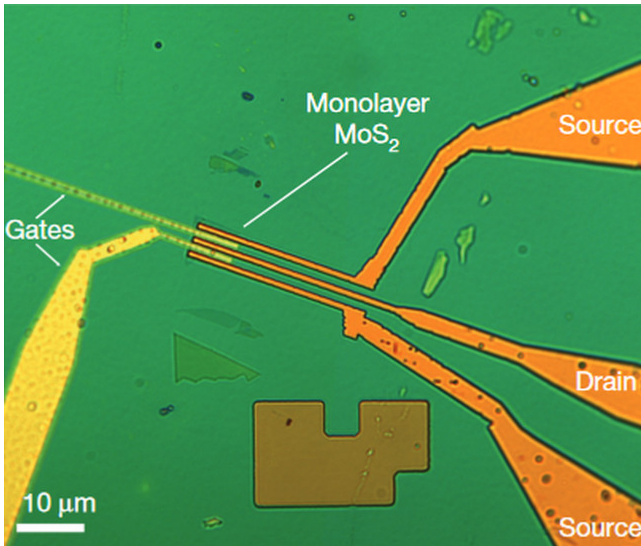
Оптическое изображение транзистора из сульфида молибдена (© EPFL)
